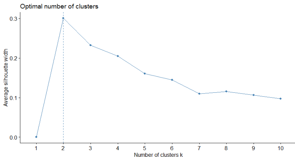
Рис. 1. График средней ширины силуэтов для выбора оптимального числа кластеров
